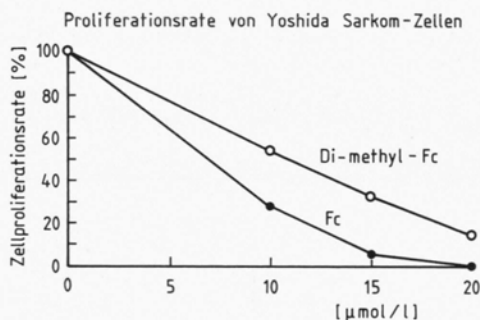
Abb. 3. Proliferationsrate von Yoshida-Sarkom-Zellen in Anwesenheit von Ferricinium- \text{BF}_4 bzw. Dimethyl-Ferricinium- \text{BF}_4 . Mittelwerte von je 4 Kultur-Röhrchen.
